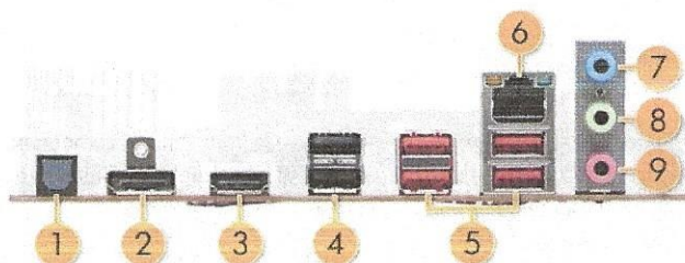
Figura 1: Pannello I/O posteriore Tampa2
